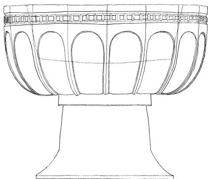
Fig. 41. Døbefont, senromansk (s. 430). 1:20. Målt og tegnet af Ejnar Mindedal Rasmussen o. 1961. – Font, Late Romanesque .
