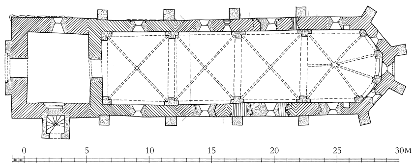
Fig. 11. Plan. 1:300. Målt af Mogens Brahde og I. Arthur-Nielsen 1963, suppleret og tegnet af Anders C. Christensen 2012. – Plan.
