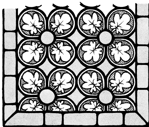
Fig. 25-26. †Glasmaleri i korets nordøstvindue (s. 421). 1:5. Målt og tegnet af Birgit Als Hansen 1963. 25. Mørtelklump med aftryk af blysprosser samt bevarede glasfragmenter. 26. Rekonstruktion af glasmaleri. – †Stained-glass in the chancel. 25. Mortar with imprint of lead mullions and fragments of glass. 26. Reconstruction of stained-glass.
