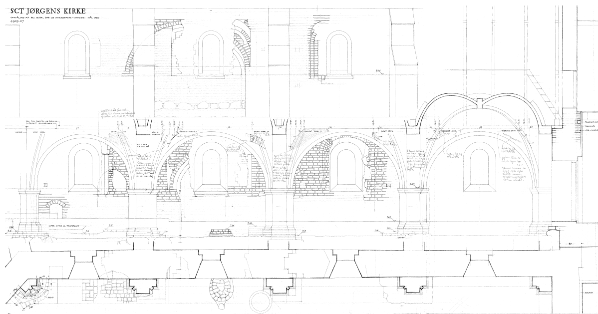
Fig. 16. Opstalter og plan af kirkens sydside. 1:150. Målt og tegnet af Ejnar Mindedal Rasmussen 1961. – Elevations and plan of the south side of the church.
