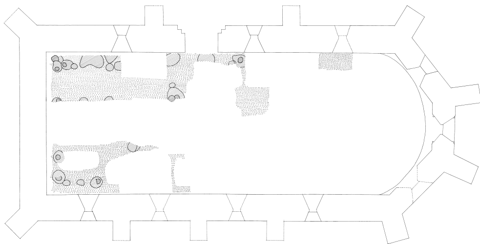
Fig. 7. Plan. 1:150. Kirkens oprindelige udstrækning med de udgravede spor af trækirken. Prikket signatur viser de områder i kirken, der er uforstyrrede af senere grave og andre nedgravninger. Stolpehullerne er skraverede, mens stolpesporene er krydsskraverede. Efter Olsen. – Plan. The original extent of the church with the excavated traces of the wooden church. Dotted areas show the places in the church that are undisturbed by later graves and other digging. The post-holes are shaded, while the traces of posts are cross-hatched.
