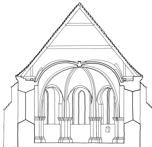
Fig. 13. Tværsnit gennem koret set mod øst. 1:150. Målt af Ejnar Mindedal Rasmussen 1962, suppleret og tegnet af Anders C. Christensen 2012. – Cross-section through nave looking east.
