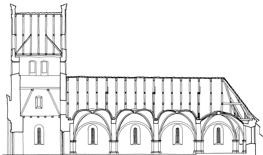
Fig. 10. Længdesnit 1:300. Målt af Ejnar Mindedal Rasmussen 1963, tegnet af Anders C. Christensen 2012. – Longitudinal section.
