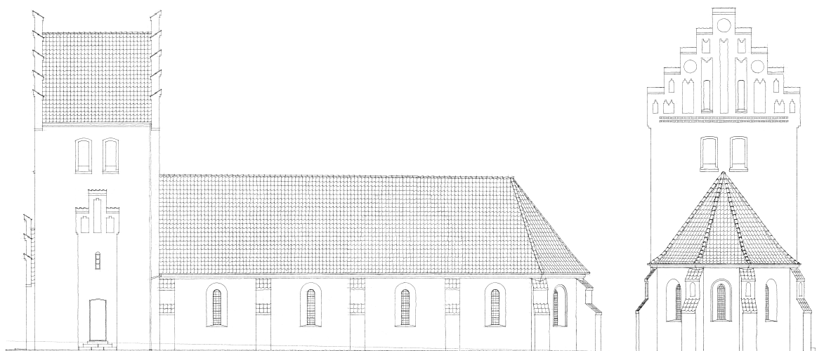
Fig. 9. Kirkens syd- og østfacade. 1:300. Målt og tegnet af Lars Mindedal Rasmussen 1995. – South and east facade of the church.
