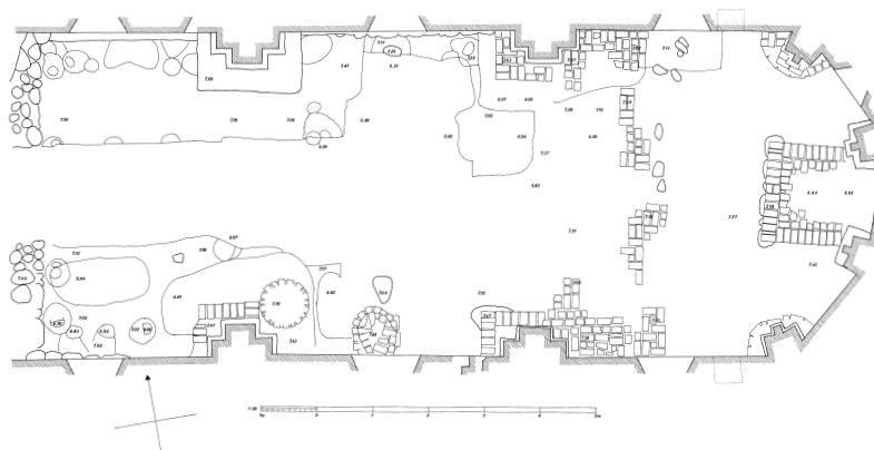
Fig. 15. Plan af kirken med rester af teglgulve (s. 419, jf. fig. 59), \dagger alterbord (s. 425) samt murede sokler til prædikestol (s. 432) og døbefont (s. 430). 1:150. Målt og tegnet af Mogens Brahde 1961. – Plan of church with remains of brick floor, Communion table and masonry foundations of pulpit.
