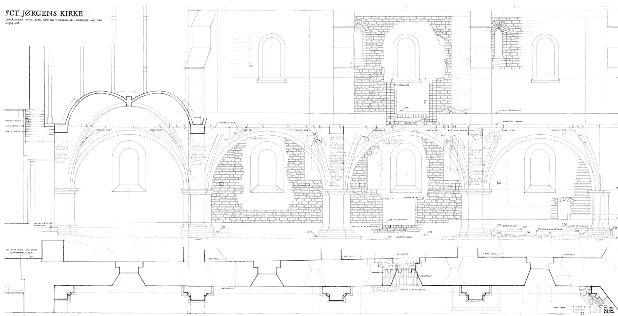
Fig. 14. Opstalter og plan af kirkens nordside. 1:150. Målt og tegnet af Ejnar Mindedal Rasmussen 1961. – Elevations and plan of the north side of the church.
