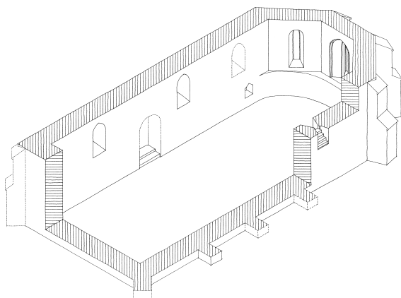
Fig. 12. Aksonometrisk rekonstruktion. 1:300. Tegnet af I. Arthur-Nielsen 1963. – Axonometric reconstruction.
