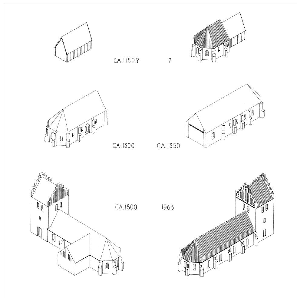
Fig. 24. Aksonometriske rekonstruktioner af kirkens bygningshistorie. 1:800. Tegnet af I. Arthur-Nielsen 1963. – Axonometric reconstructions of the construction history of the church.
